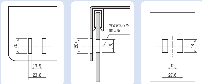
フラップロック(オス)
